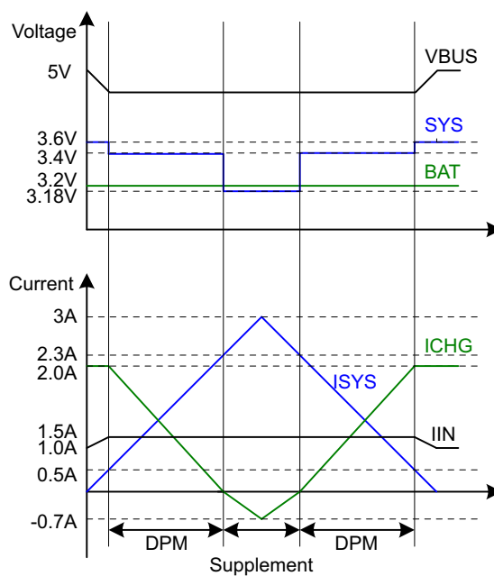
图 12. DPM Response
