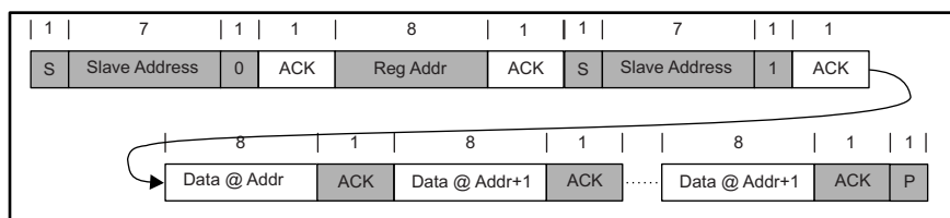
图 26. Multi-Read
