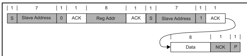
图 24. Single Read
