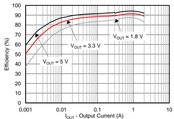
Tps562200 效率
