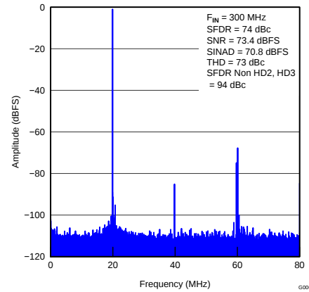
图 11. FFT for 300-MHz Input Signal ( 2.5\text{-V}_{\text{PP}} Full-Scale)
