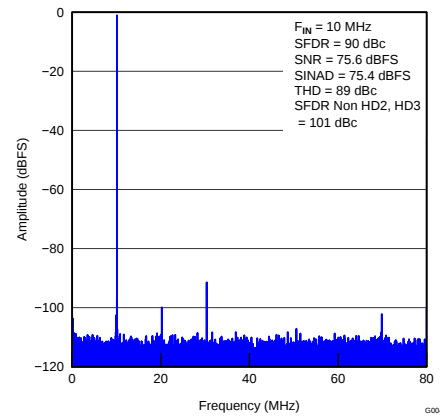
图 9. FFT for 10-MHz Input Signal ( 2.5\text{-V}_{\text{PP}} Full-Scale)
