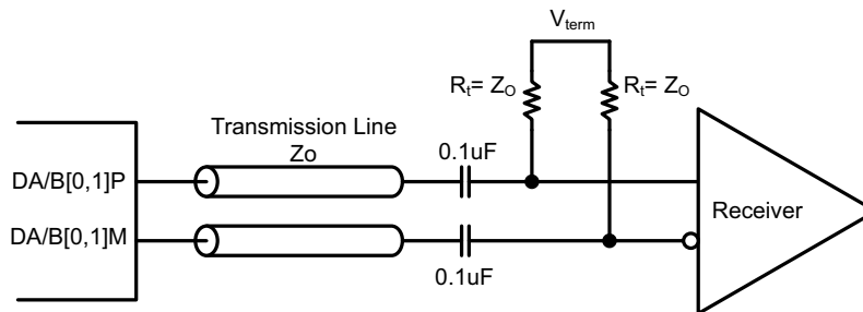
图 49. CML Output Connections
