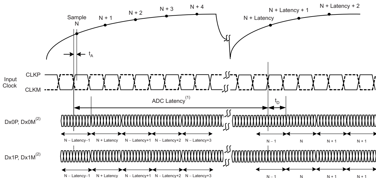
图 3. ADC Latency
