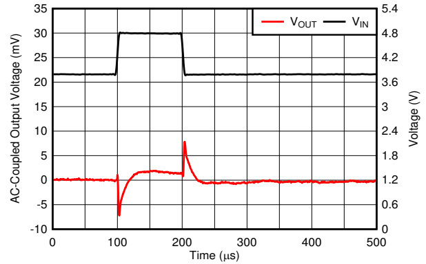
图 6-38. Line Transient
