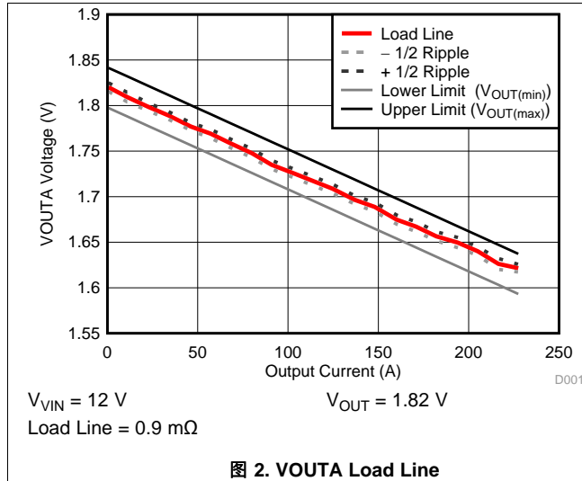
图 2. VOUTA Load Line
