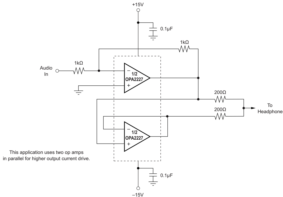
图 48. 耳机放大器
