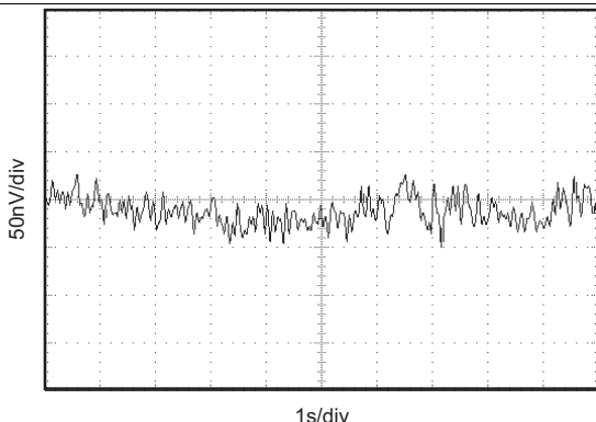
图 7. 输入噪声电压与时间的关系
