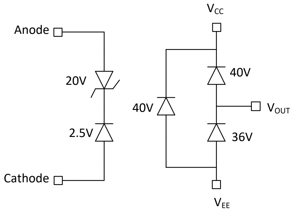
图 24. ESD Structure
