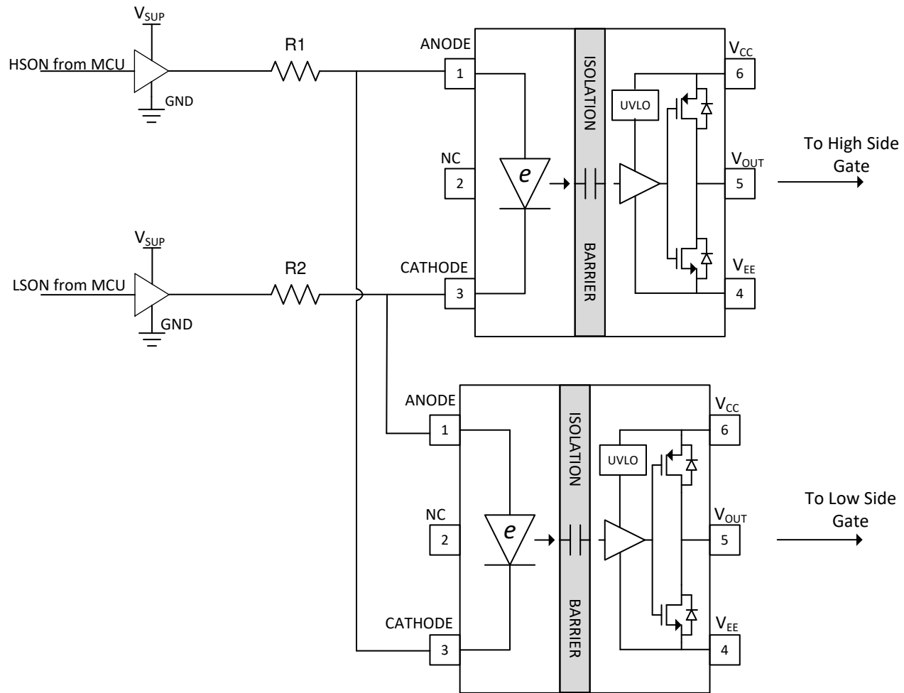
图 21. Interlock
