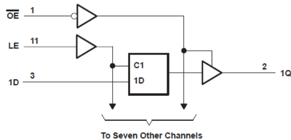
功能方框图
