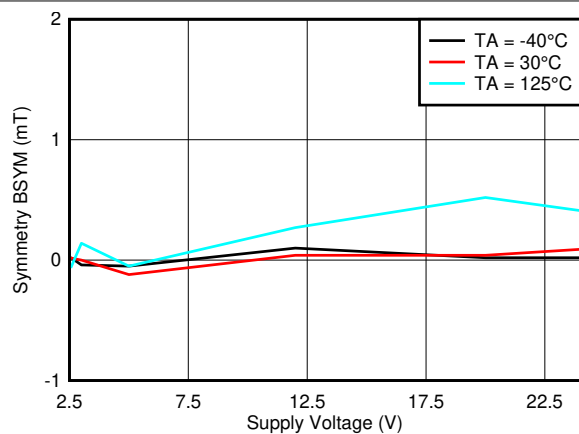
图 7-21. B_{SYM(x)} vs. V_{CC}
