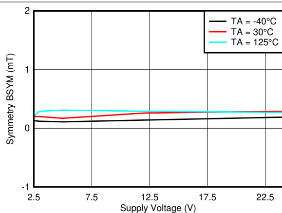
图 7-23. B_{SYM(y)} vs. V_{CC}
