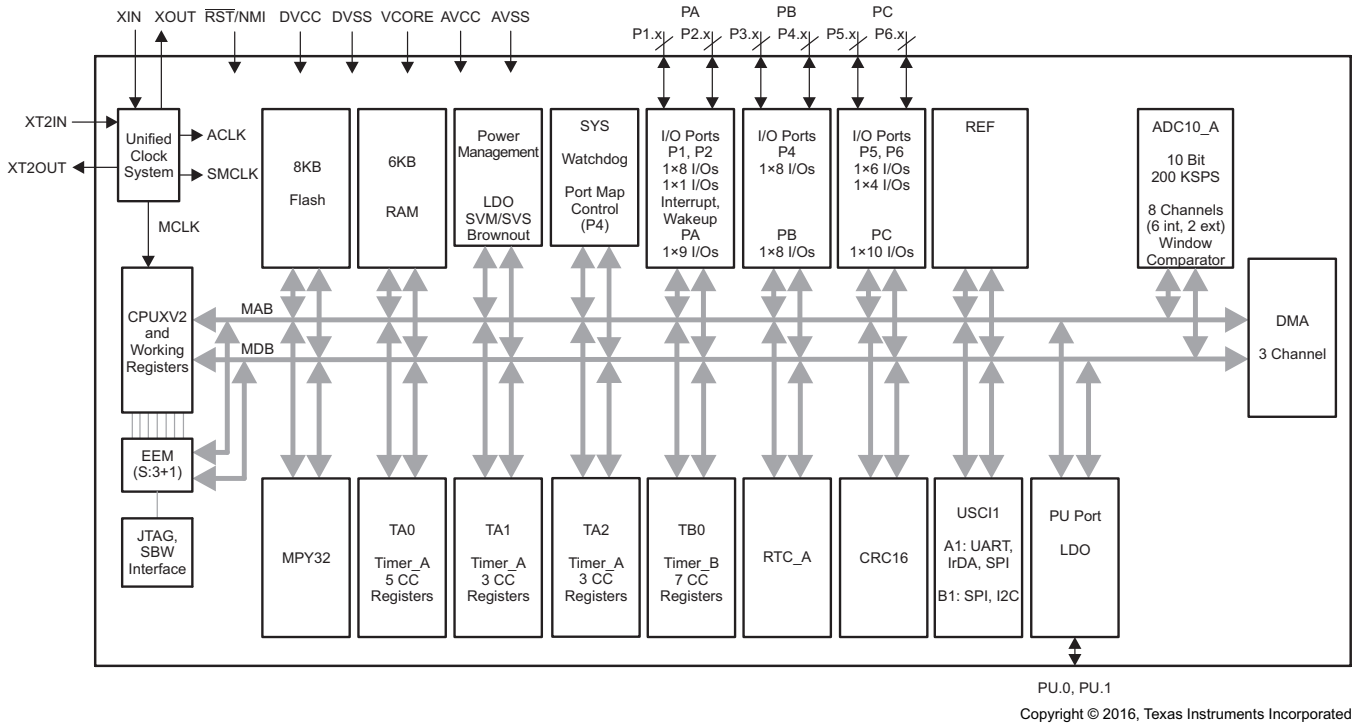
图 1-3. 功能方框图 – MSP430F5304IRGZ、MSP430F5304IPT
