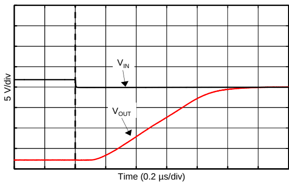
图 27. 无相位反转
