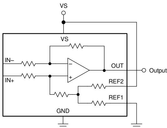
图 8-6. Midsupply Voltage Output
