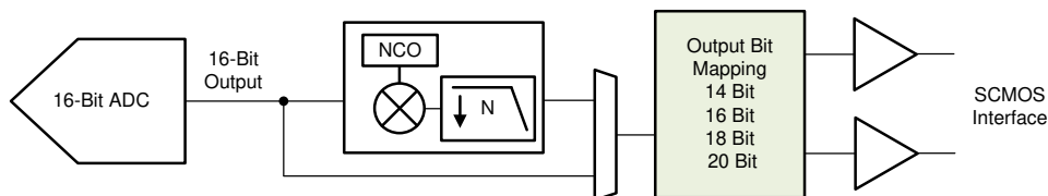
图 8-37. Interface output bit mapper
