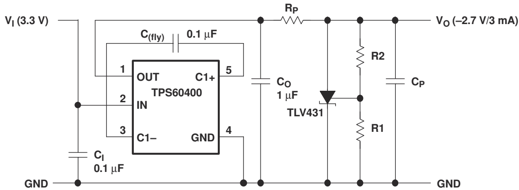
图 9-11. GaAs Supply
