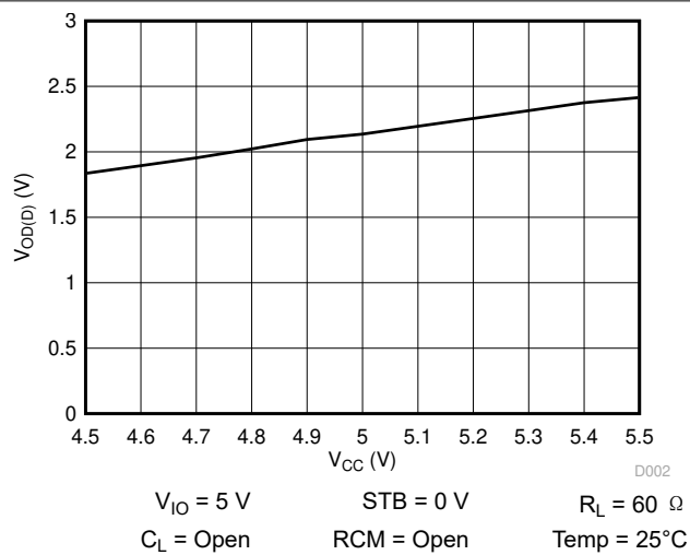
图 7-2. V_{OD(D)} over V_{CC}
