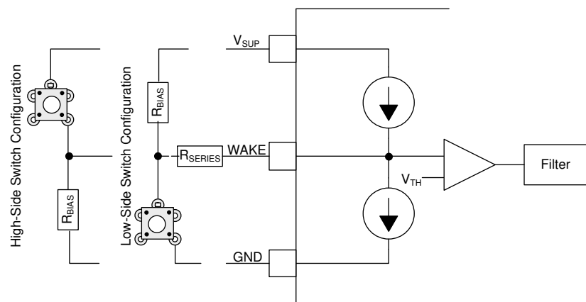
图 9-6. TCAN1043xx-Q1 WAKE Circuit Example
