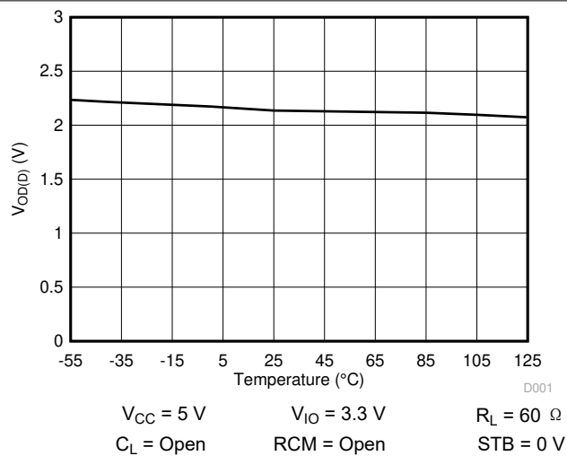
图 7-1. V_{OD(D)} over Temperature
