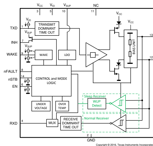
功能模块图
