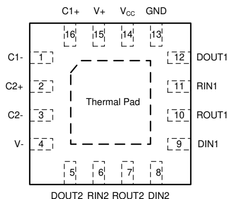
图 5-2. RGT package, 16 Pin VQFN, Top View
