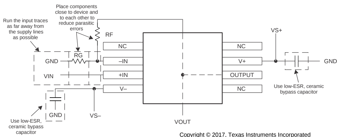
图 33. 布局建议
