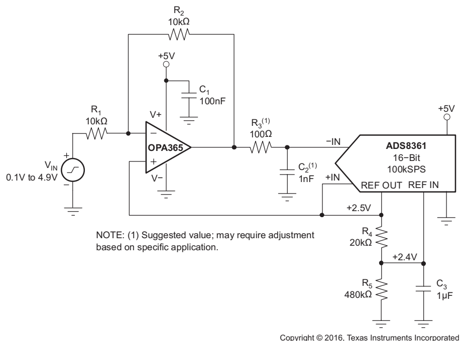
图 31. 驱动 ADS8361
