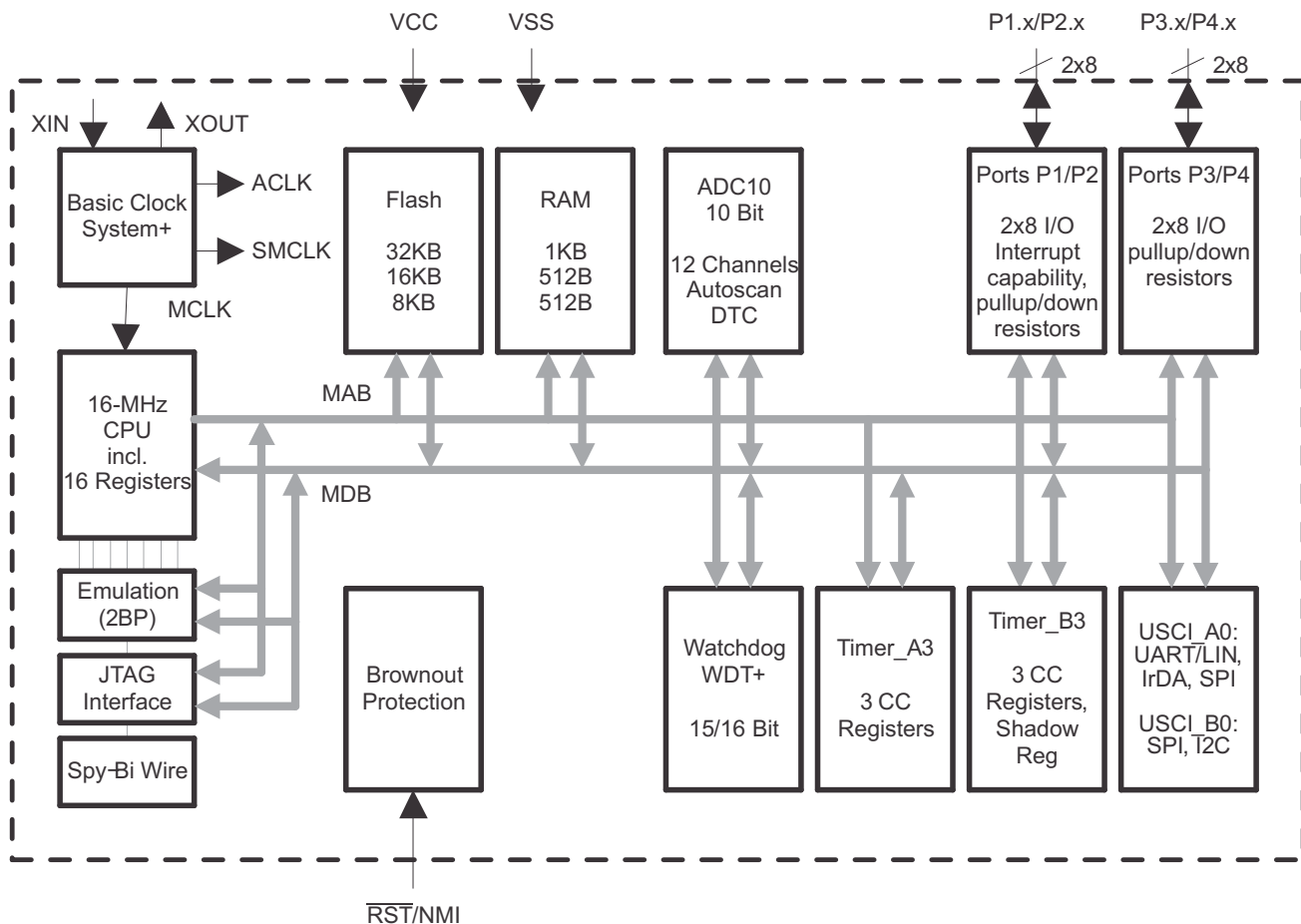
图 1-1. 功能方框图
