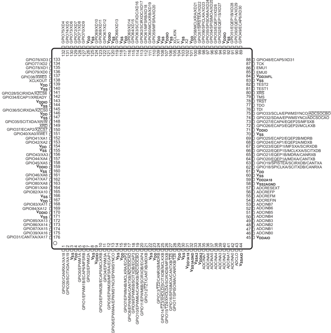
图 6-1. F2833x, F2823x 176-Pin PGF/PTP LQFP (Top View)
