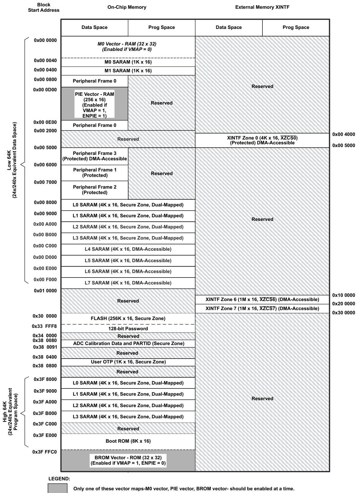
图 8-23. F28335, F28333, F28235 Memory Map
