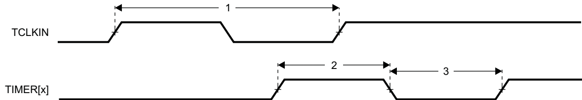
图 7-2. Timer Timing
