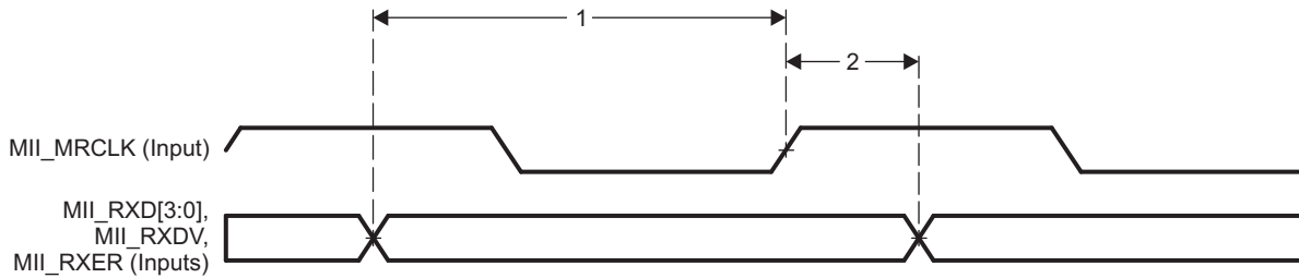
图 5-128. PRU-ICSS MII_RXD[3:0], MII_RXDV, and MII_RXER Timing
