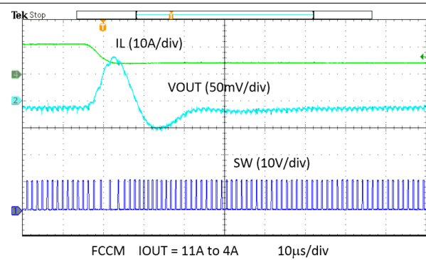
图 8-25. Unload Transient
