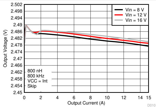
图 8-7. Output Voltage vs Output Current
