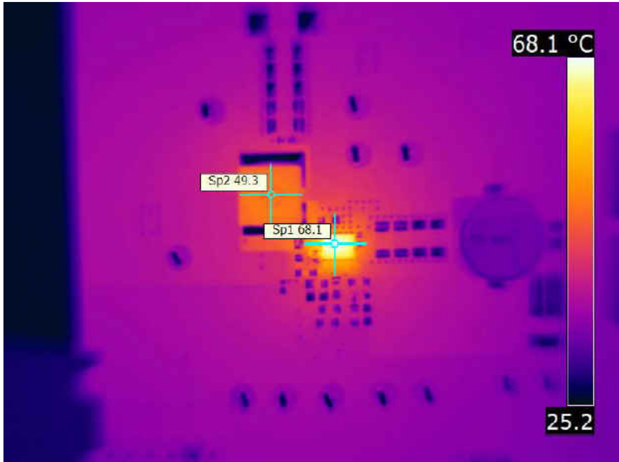
图 10-2. Thermal Image At 25°C Ambient
