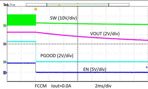
图 8-17. Enable Power Down Iout = 0 A
