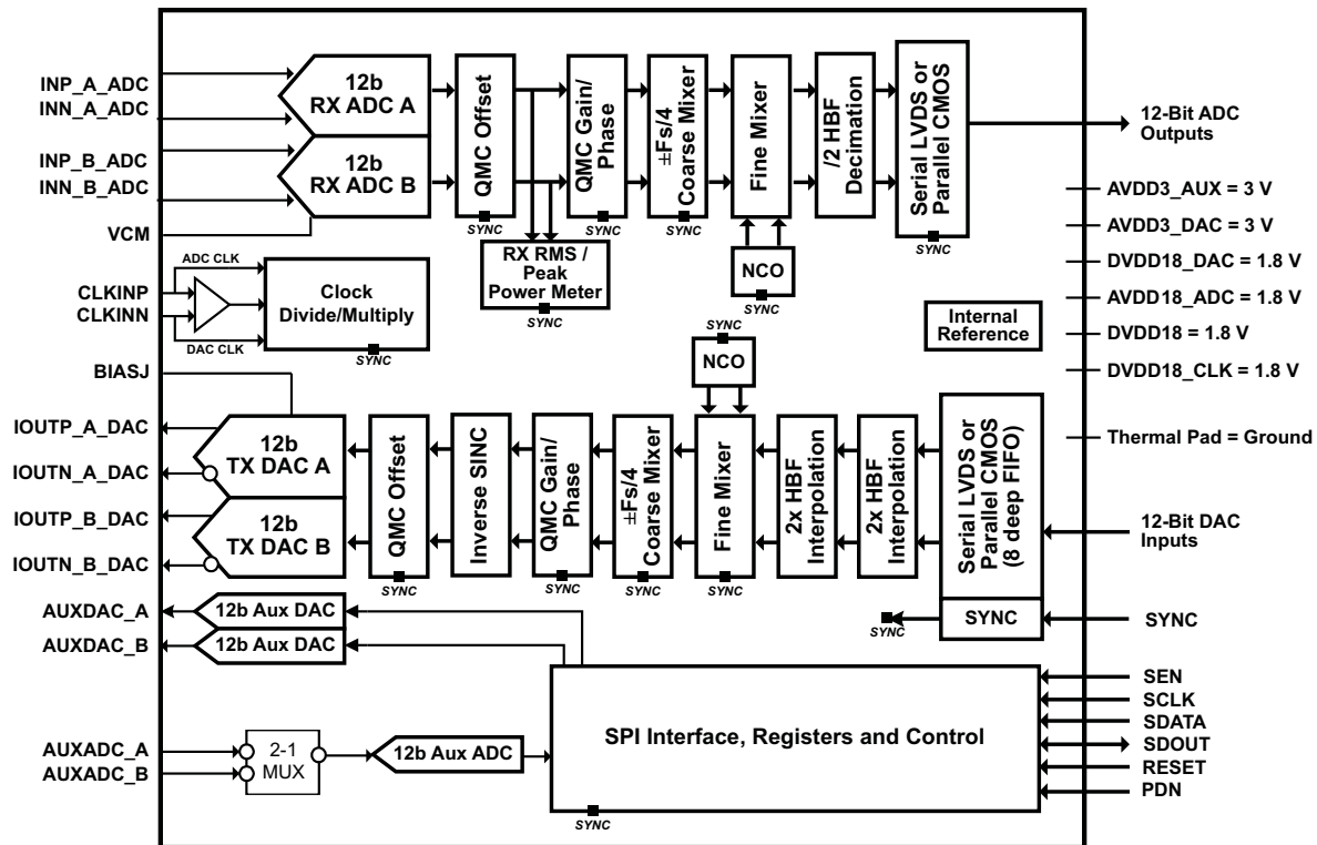
图 1-1. AFE7222/AFE7225 的方框图
