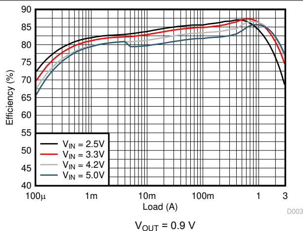
图 9-7. Efficiency
