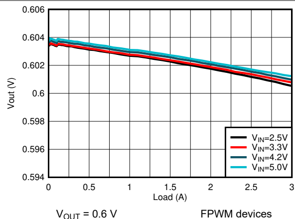
图 9-6. Load Regulation
