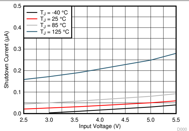
图 7-4. Shutdown Current
