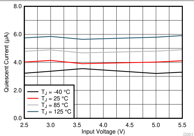
图 7-3. Quiescent Current
