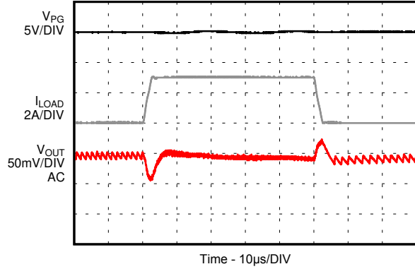
图 9-33. Load Transient
