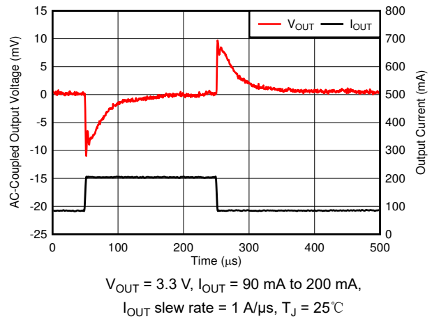
图 6-62. Load Transient
