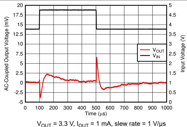
图 6-24. Line Transient
