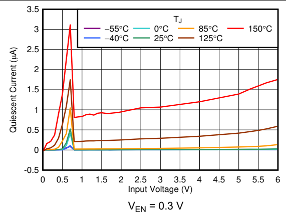
图 6-18. I_{SHDN} vs V_{IN}
