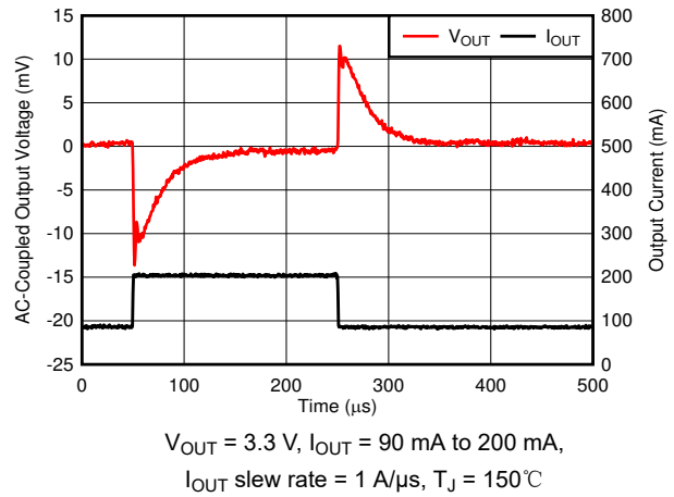
图 6-64. Load Transient
