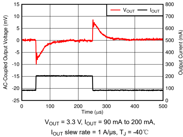
图 6-63. Load Transient
