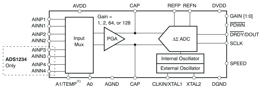
方框图
