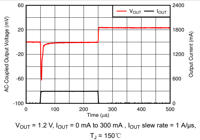
图 6-52. Load Transient
