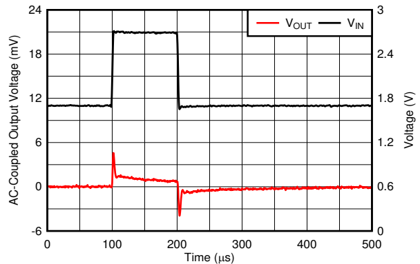
图 6-26. Line Transient
