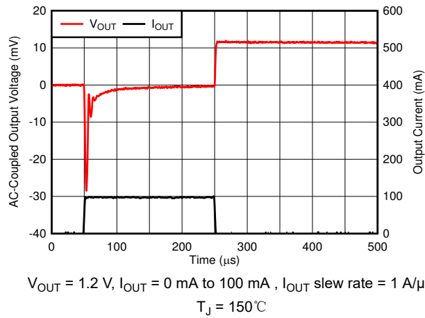
图 6-49. Load Transient
