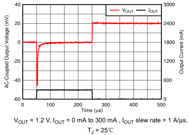
图 6-50. Load Transient
