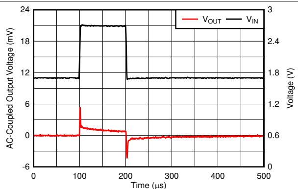
图 6-28. Line Transient
