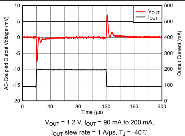
图 6-54. Load Transient
