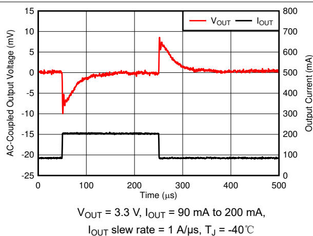
图 6-63. Load Transient
