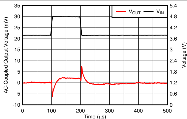
图 6-38. Line Transient
