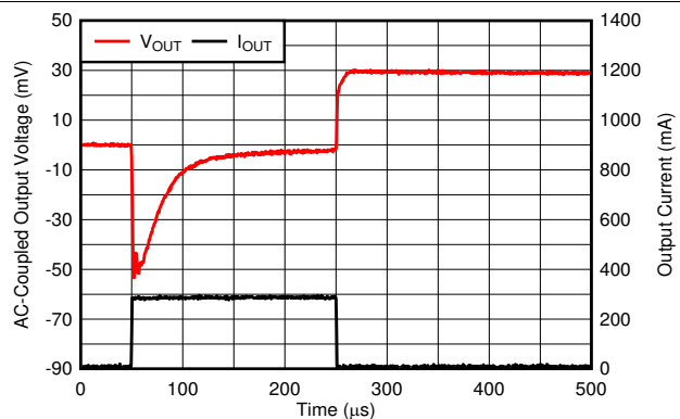
图 6-57. Load Transient
