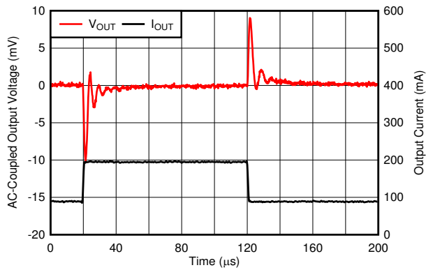
图 6-55. Load Transient
