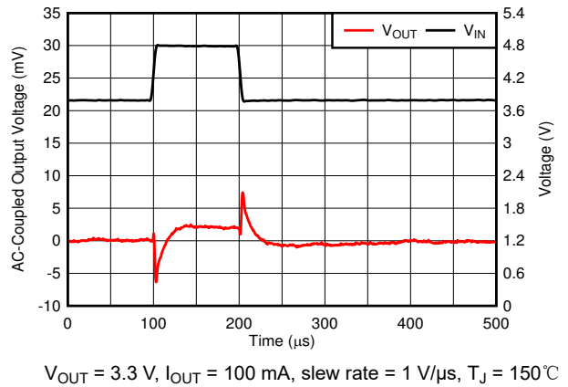
图 6-40. Line Transient
