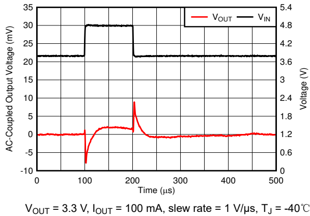
图 6-39. Line Transient
