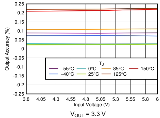
图 6-4. Output Accuracy vs V_{\text{IN}}
