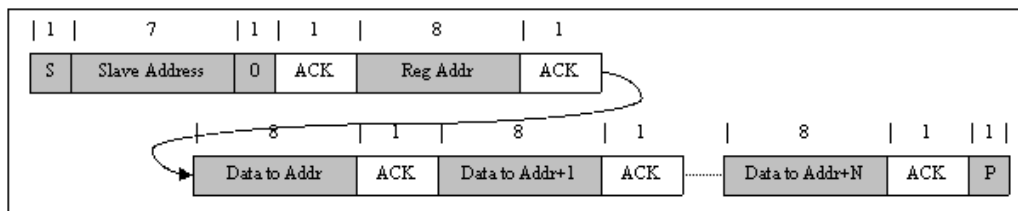
图 21. Multi Write
