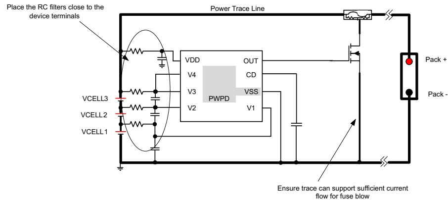
图 11-1. Layout Example
