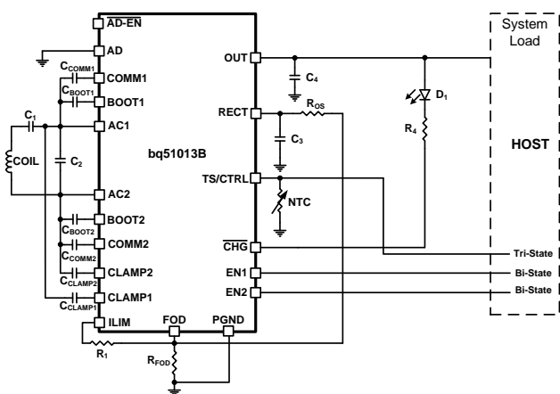
简化原理图
