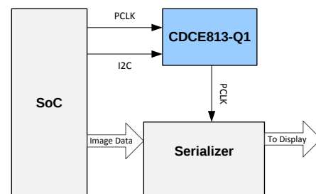
典型应用原理图
