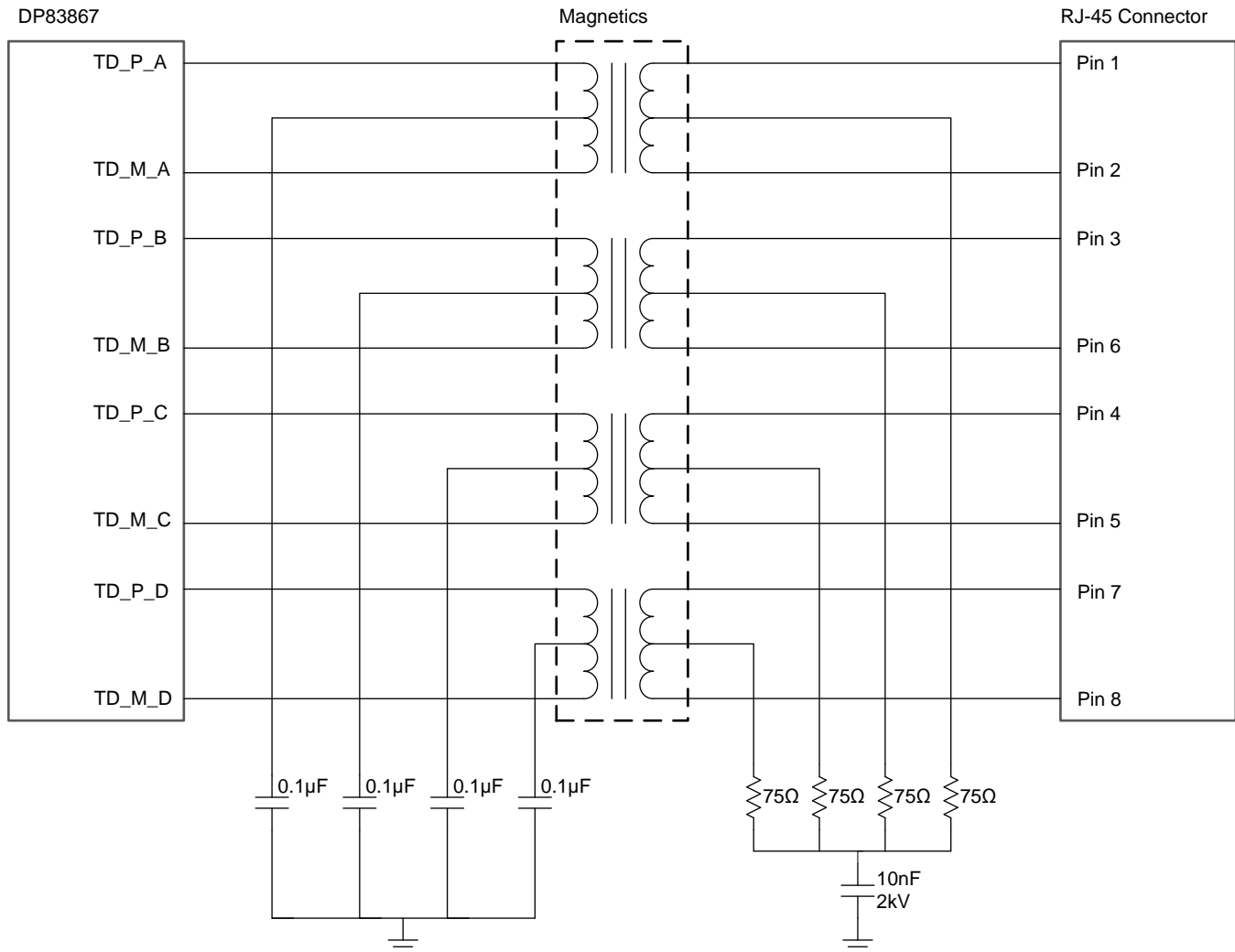
图 30. Magnetics Connections
