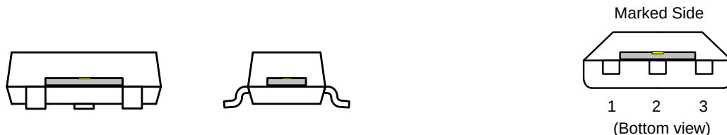
图 25. SOT-23 (DBZ) 封装
