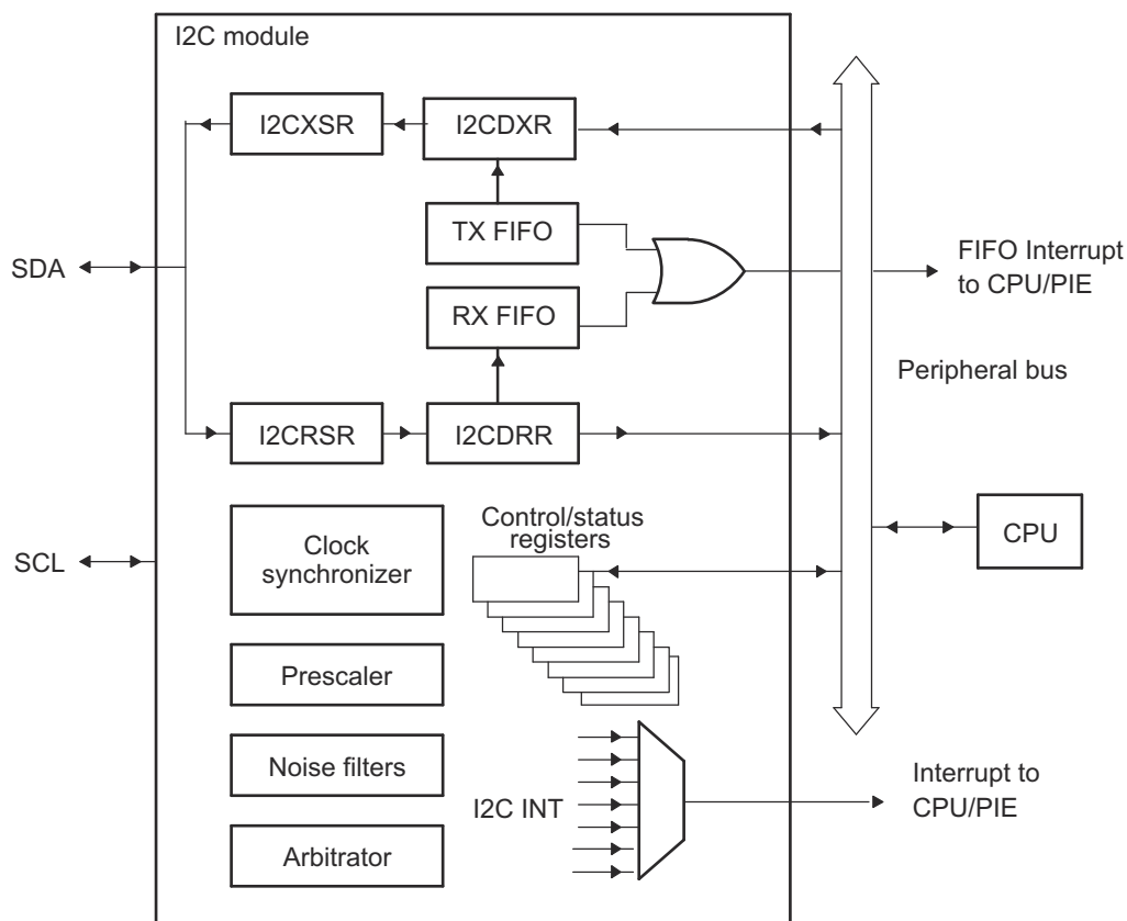
图 7-70. I2C Peripheral Module Interfaces
