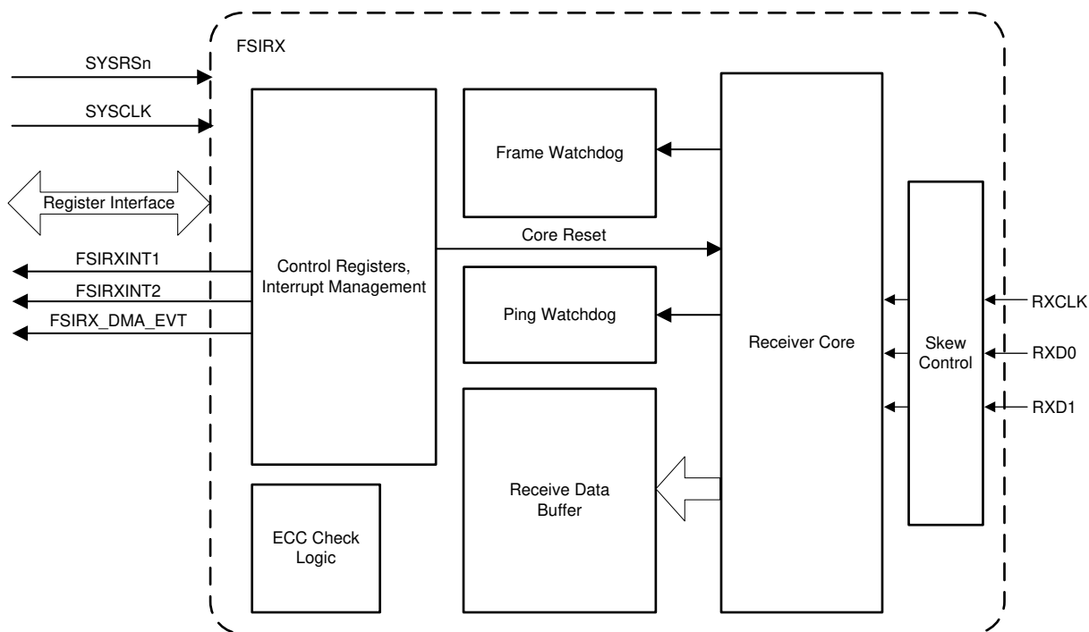
图 7-88. FSIRX Block Diagram
