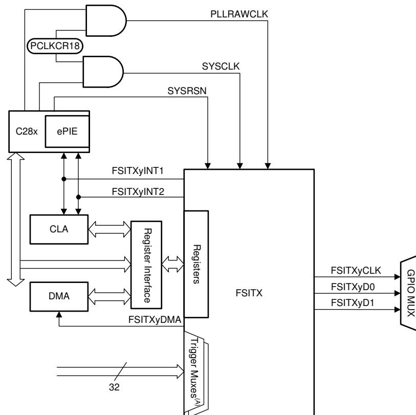
图 7-84. FSITX CPU Interface
