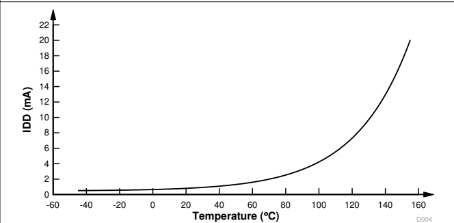
图 7-5. Halt Current Versus Temperature (°C)
