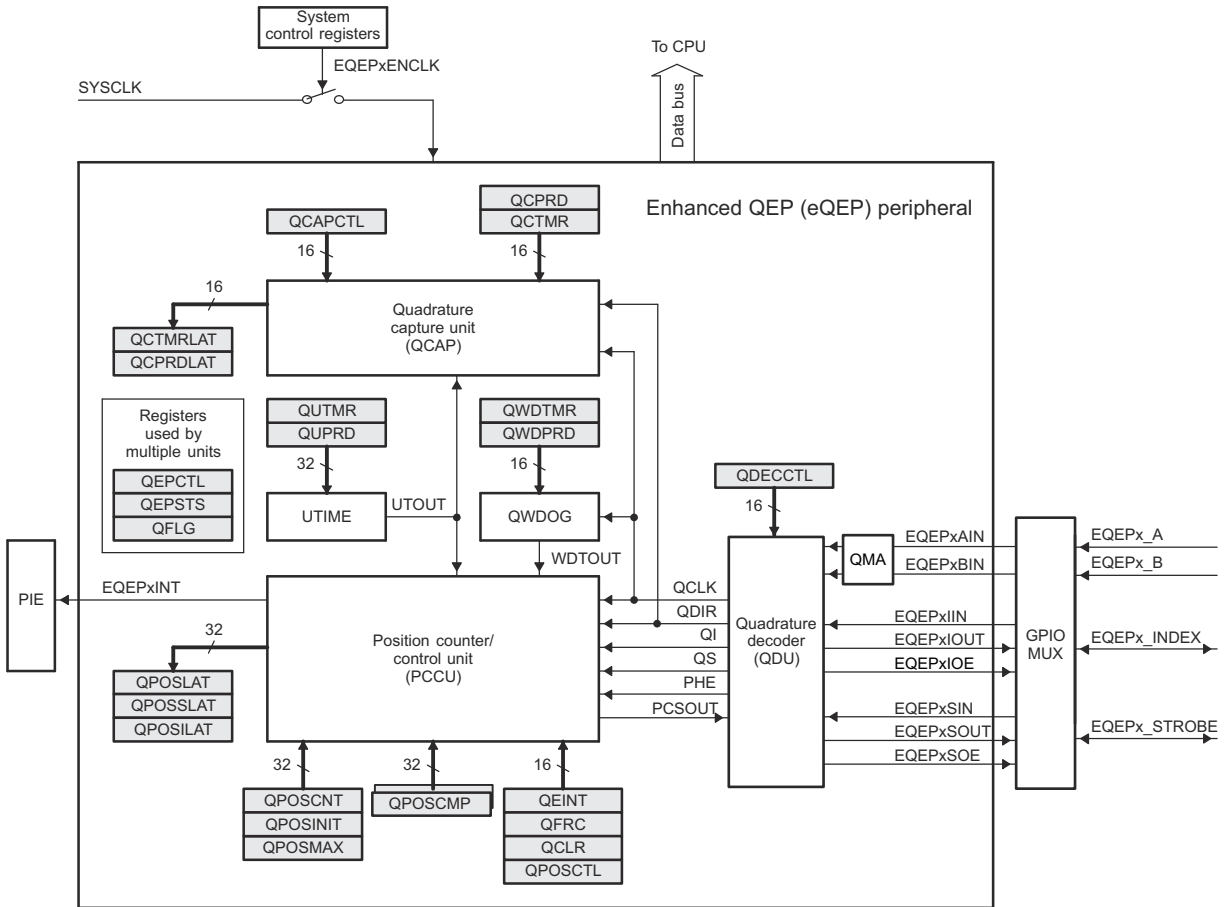
图 7-63. eQEP Block Diagram
