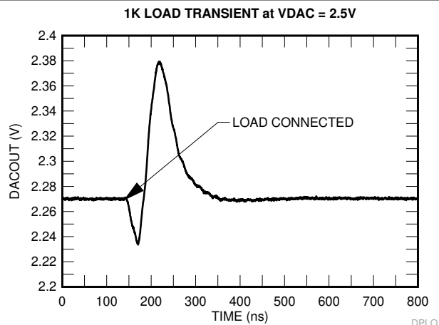
图 7-46. 1-k \Omega Load Transient
