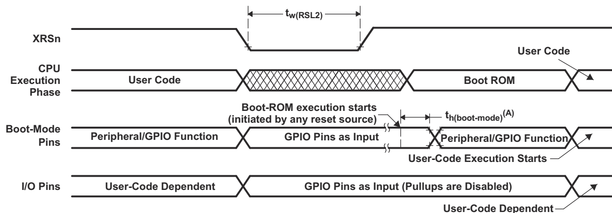
图 7-9. Warm Reset
