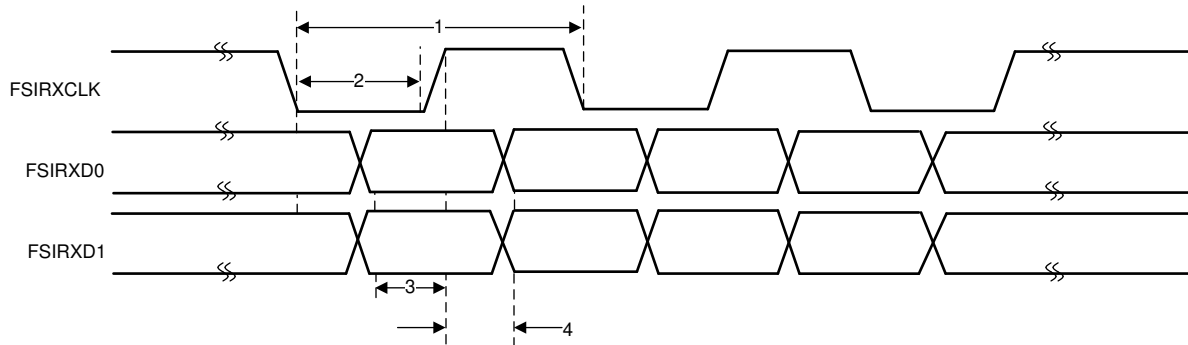
图 7-89. FSIRX Timings
