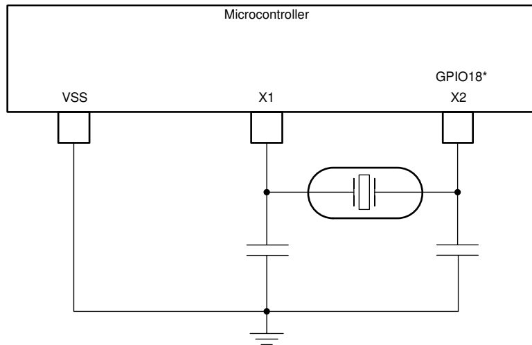
图 7-13. External Crystal
