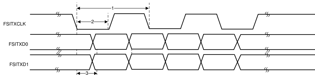
图 7-86. FSITX Timings
