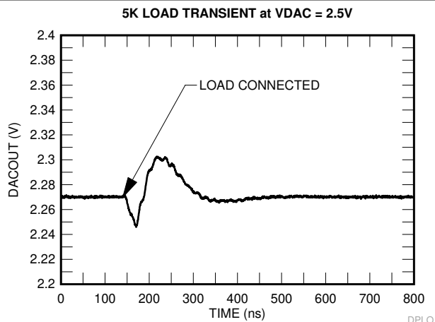
图 7-47. 5-k \Omega Load Transient
