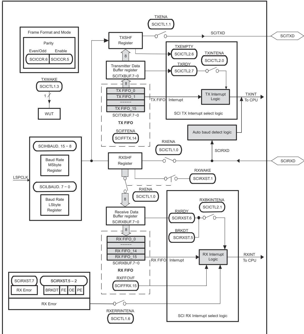
图 7-73. SCI Block Diagram
