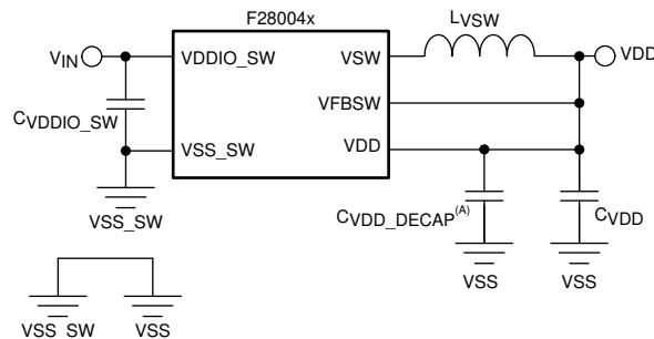
图 7-6. DC-DC Circuit Schematic
