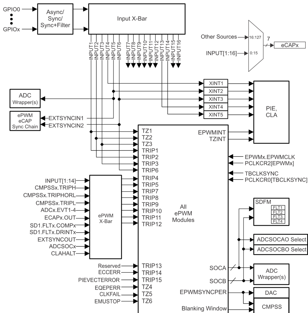
图 7-59. ePWM Trip Input Connectivity
