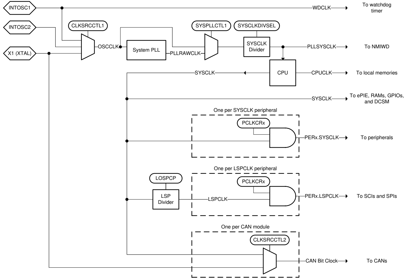
图 7-10. Clocking System
