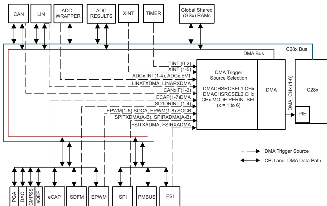
图 8-3. DMA Block Diagram
