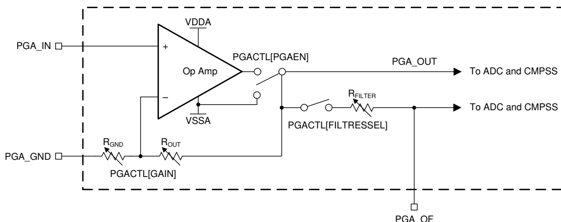
图 7-36. PGA Block Diagram
