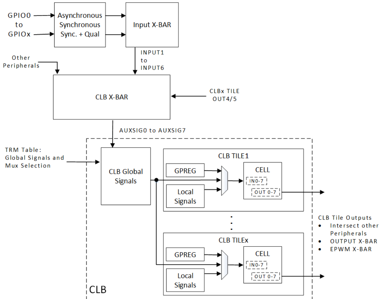
图 8-5. CLB Overview
