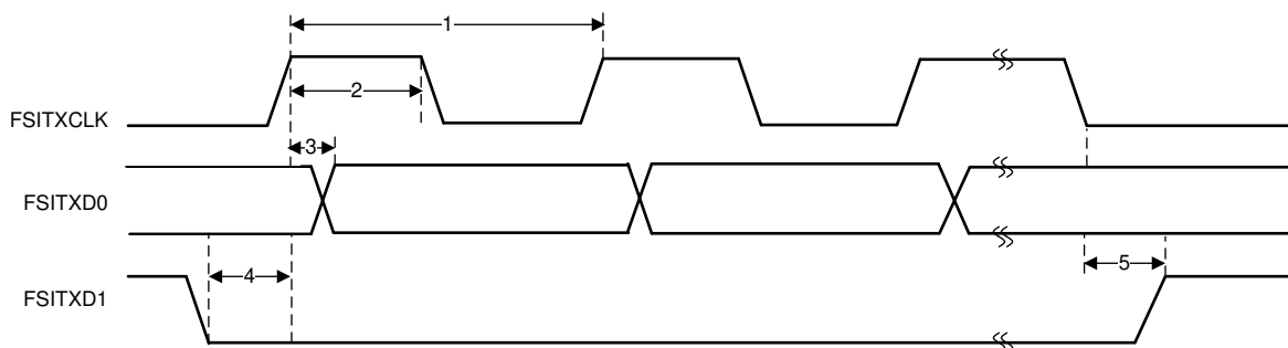
图 7-90. FSITX SPI Signaling Mode Timings
