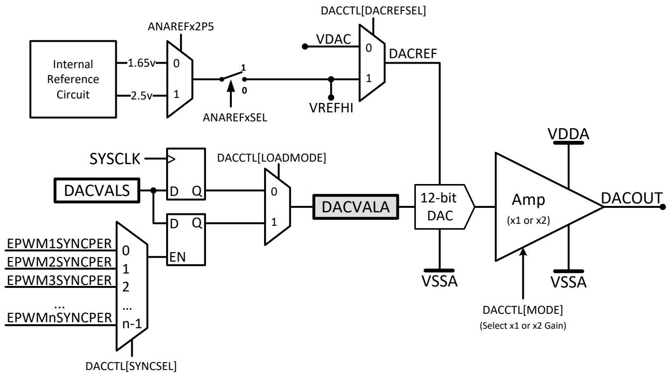
图 7-38. DAC Module Block Diagram
