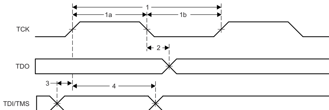
图 7-19. JTAG Timing
