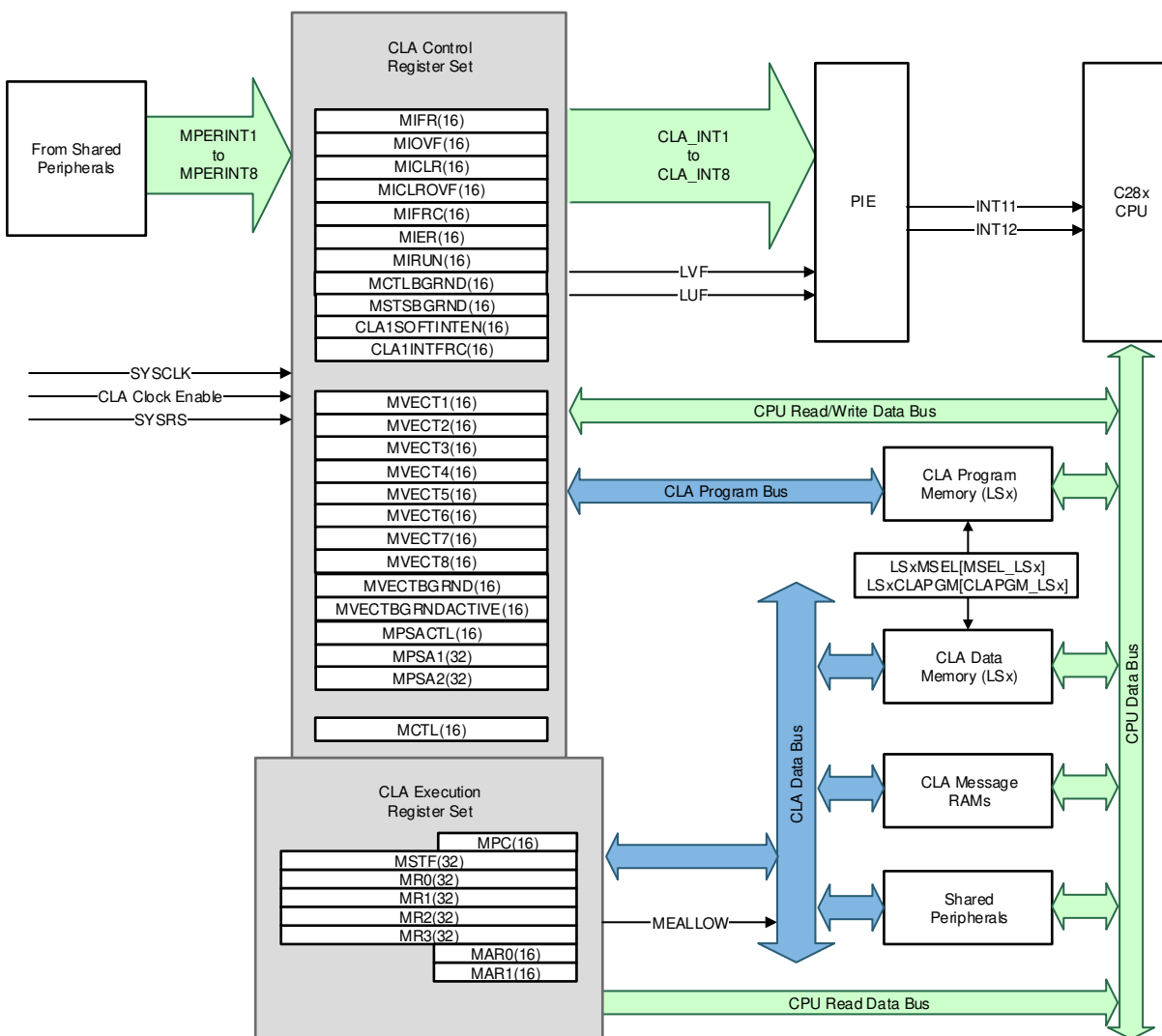
图 8-2. CLA Block Diagram
