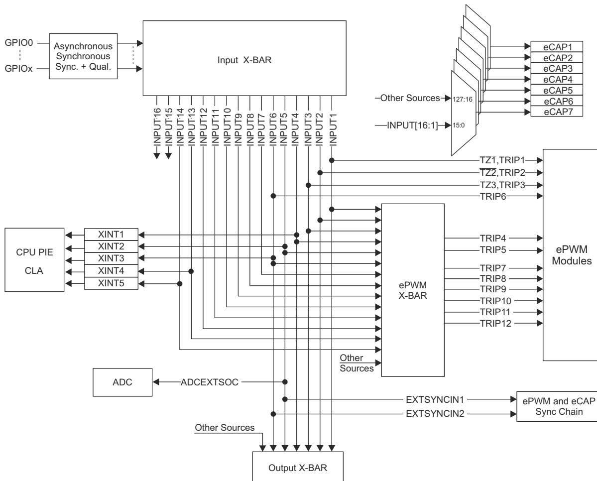
图 6-5. Input X-BAR
