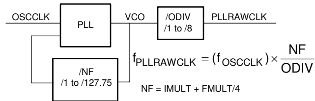
图 7-11. System PLL
