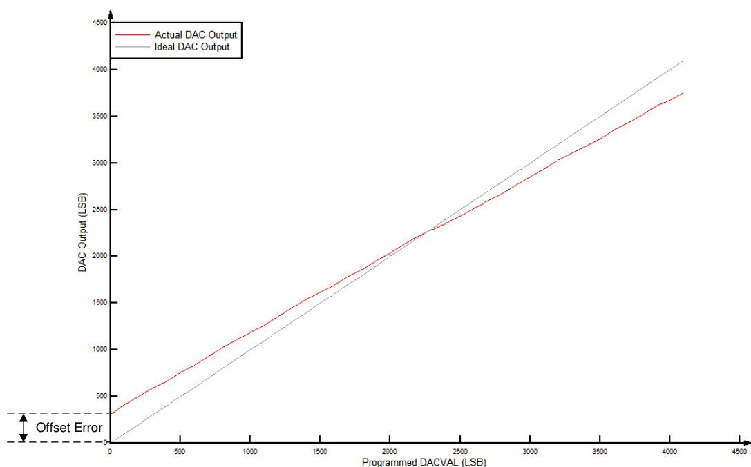
图 7-51. CMPSS DAC Static Offset
