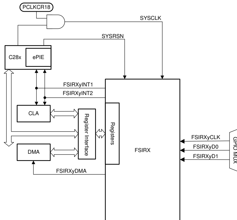
图 7-87. FSIRX CPU Interface
