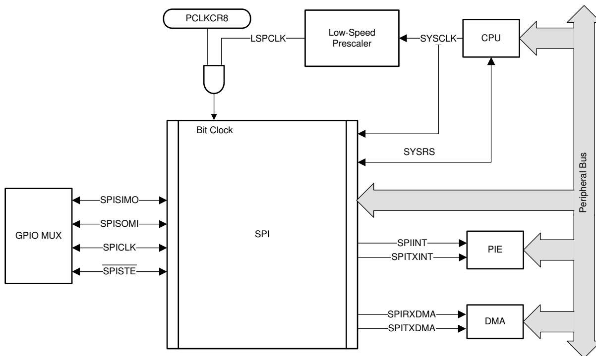
图 7-74. SPI CPU Interface
