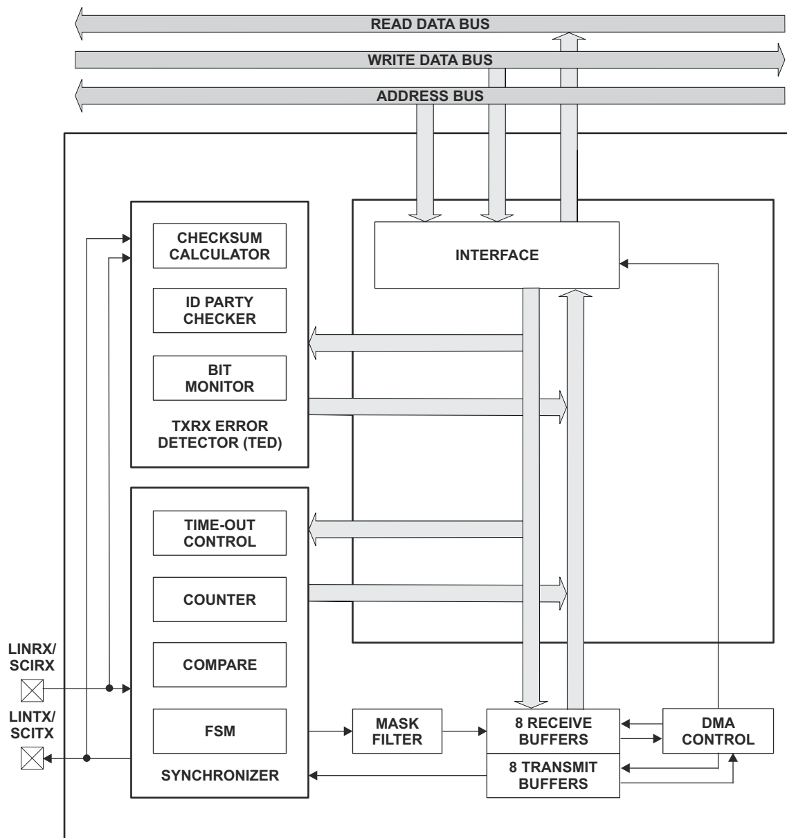
图 7-83. LIN Block Diagram
