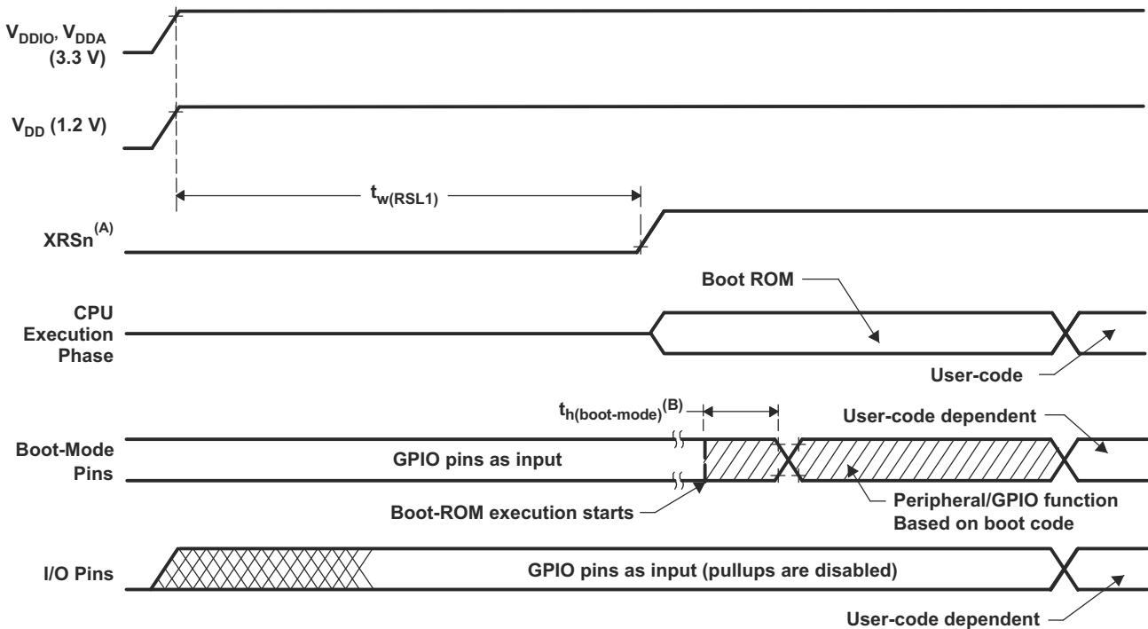
图 7-8. Power-on Reset
