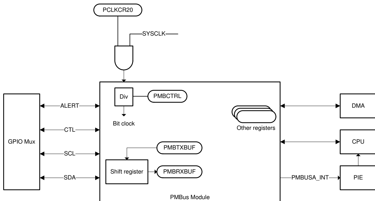
图 7-72. PMBus Block Diagram
