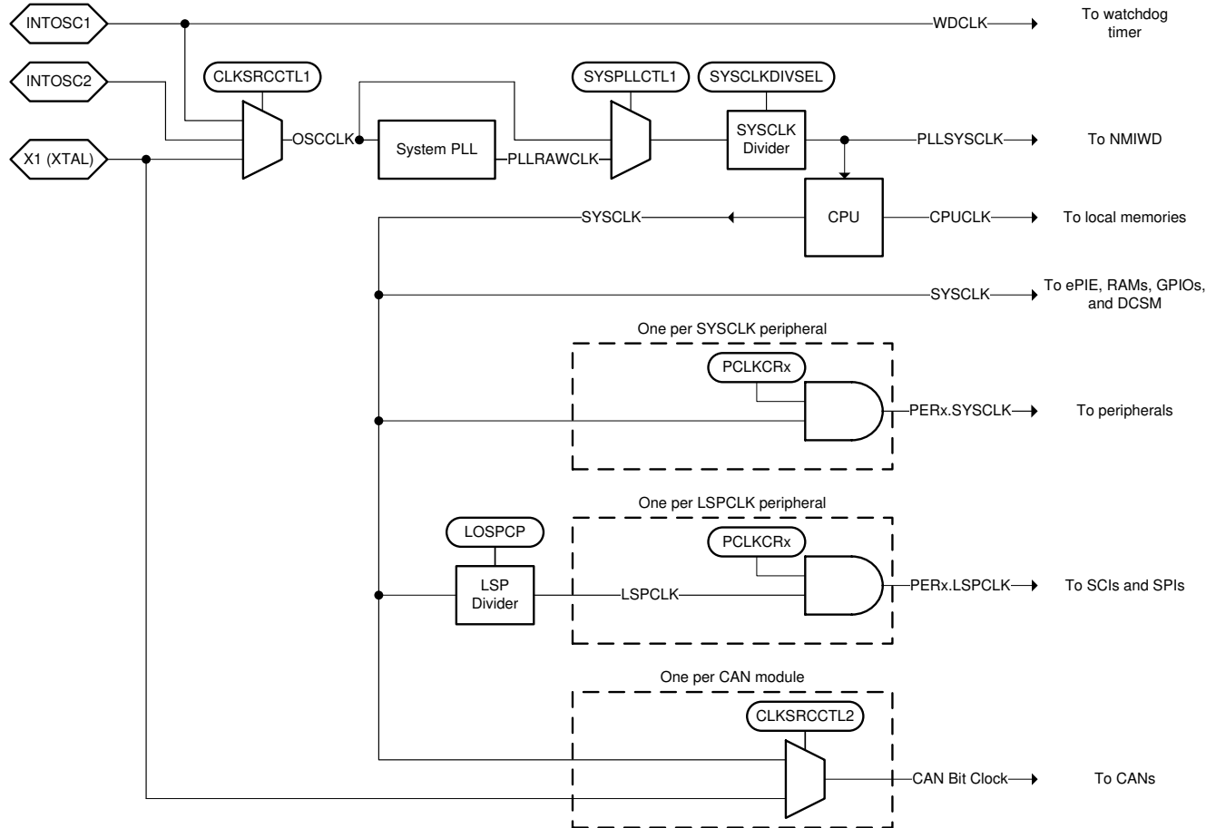
图 7-10. Clocking System
