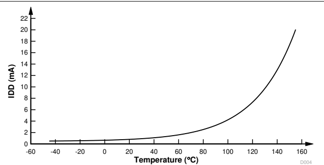
图 7-5. Halt Current Versus Temperature (°C)
