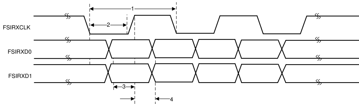
图 7-89. FSIRX Timings
