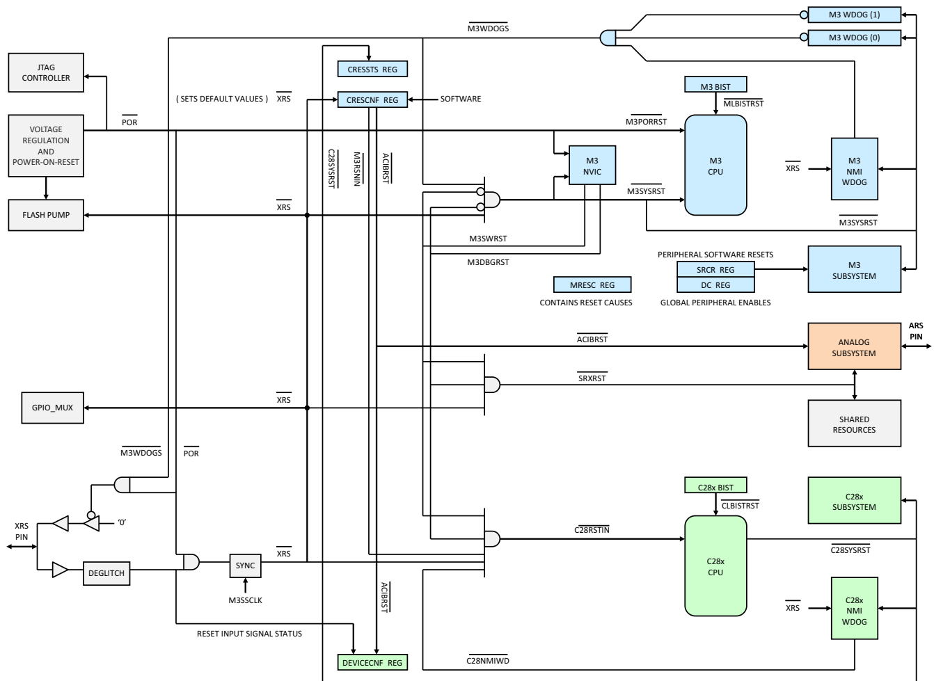
图 8-5. Resets
