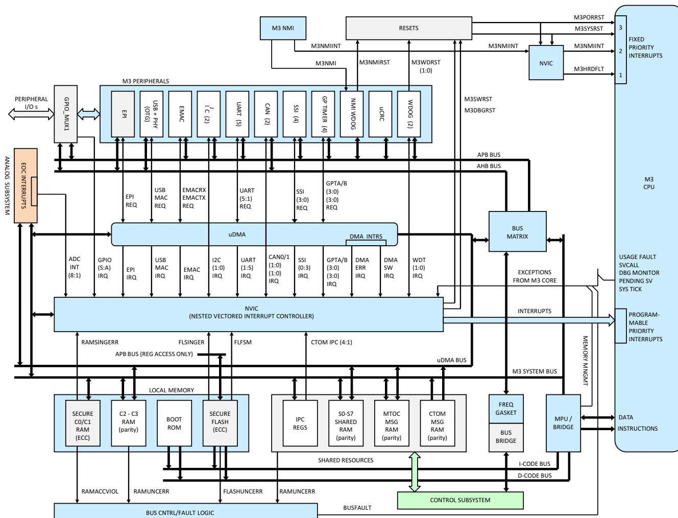
图 8-1. Master Subsystem
