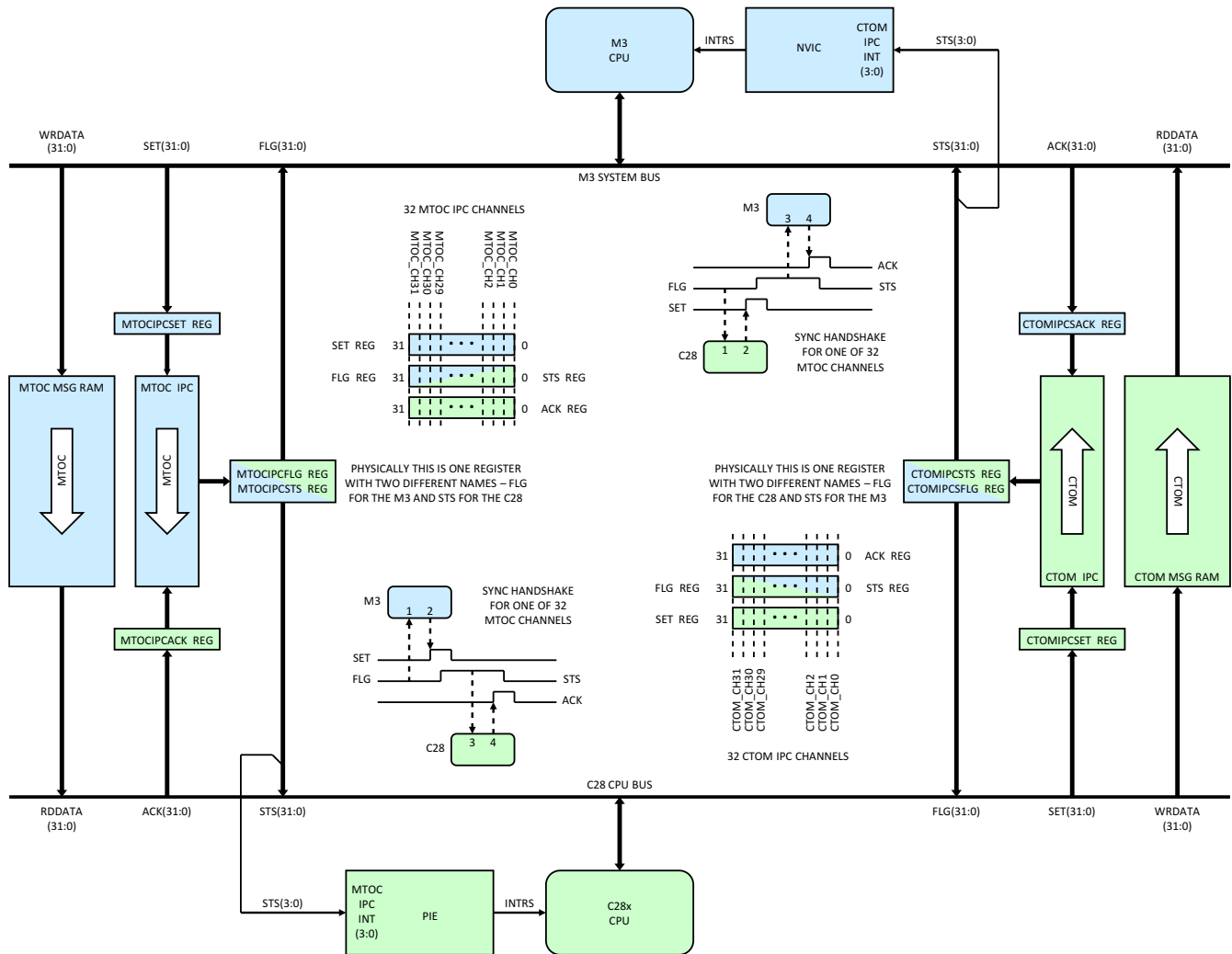
图 7-15. IPC
