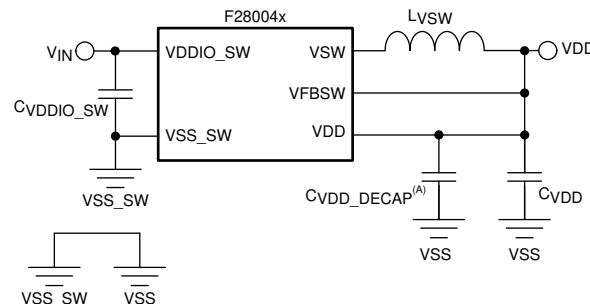
图 7-6. DC-DC Circuit Schematic
