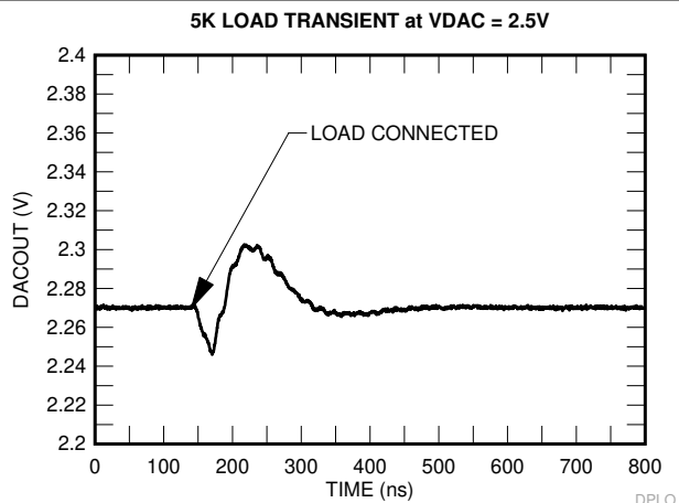
图 7-47. 5-k \Omega Load Transient
