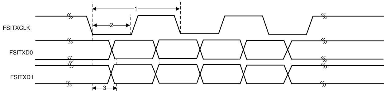
图 7-86. FSITX Timings
