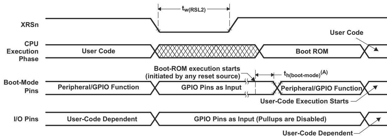
图 7-9. Warm Reset
