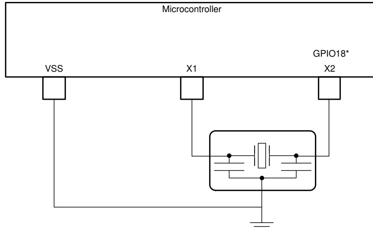
图 7-14. External Resonator
