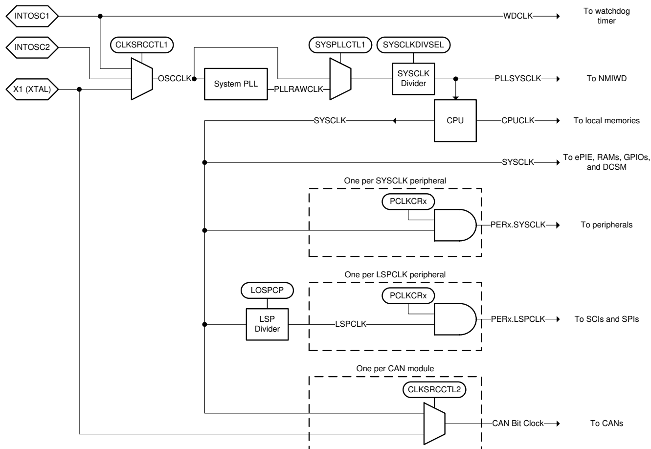
图 7-10. Clocking System
