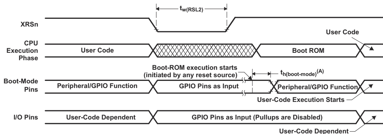
图 7-9. Warm Reset
