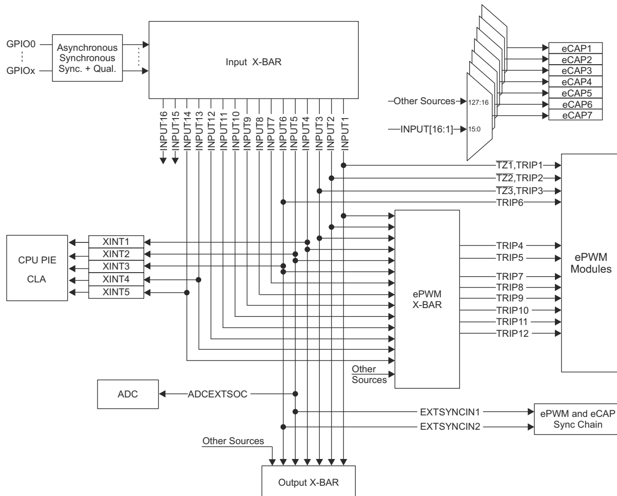
图 6-5. Input X-BAR
