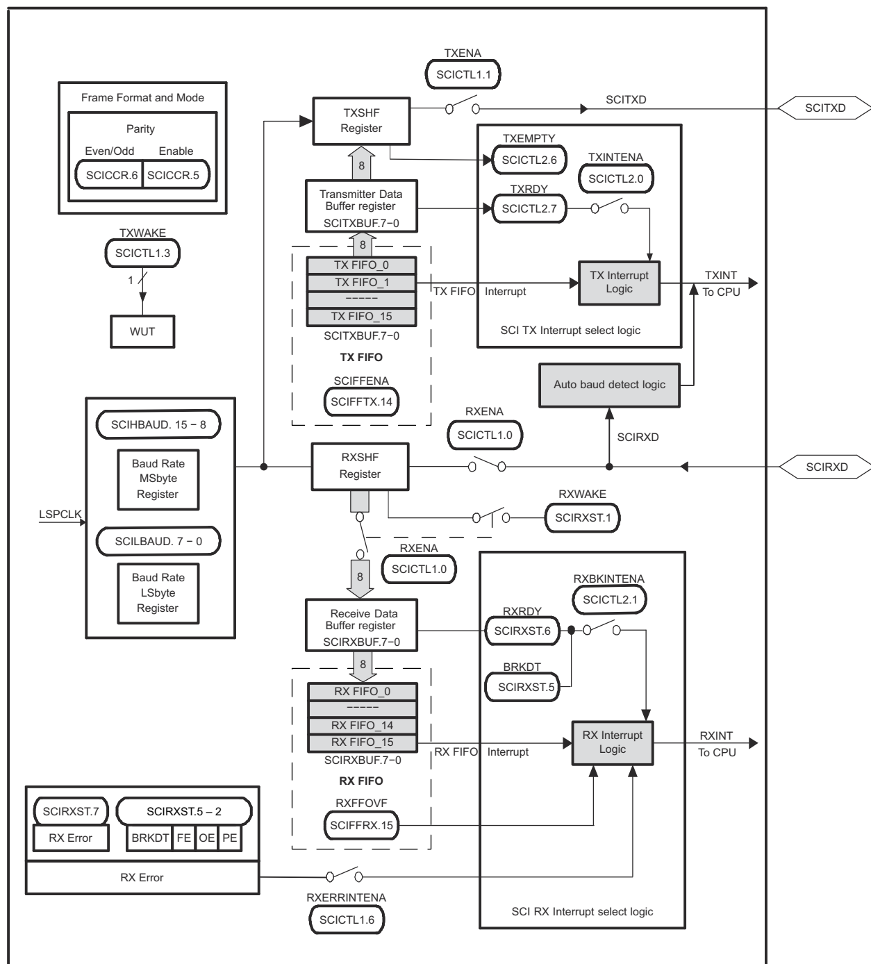
图 7-73. SCI Block Diagram
