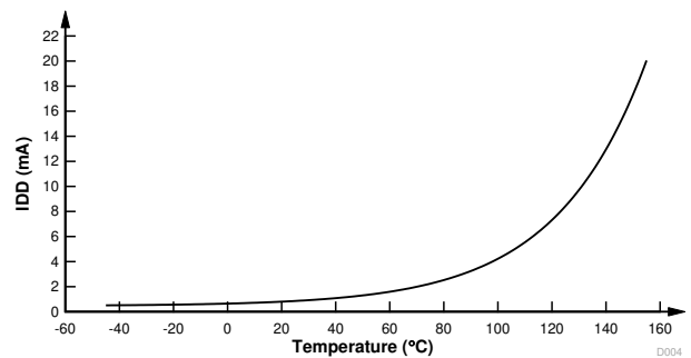
图 7-5. Halt Current Versus Temperature (°C)
