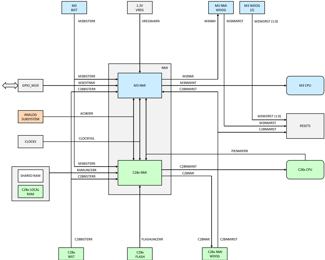
图 8-4. Cortex-M3 NMI and C28x NMI
