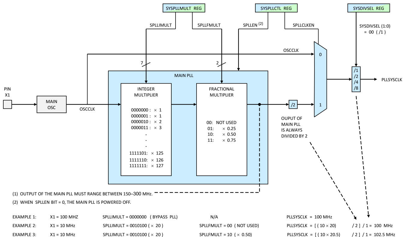
图 8-8. Main PLL
