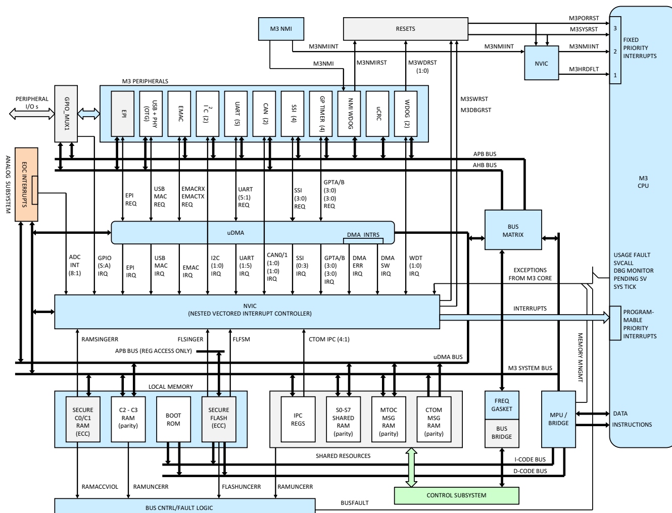
图 8-1. Master Subsystem
