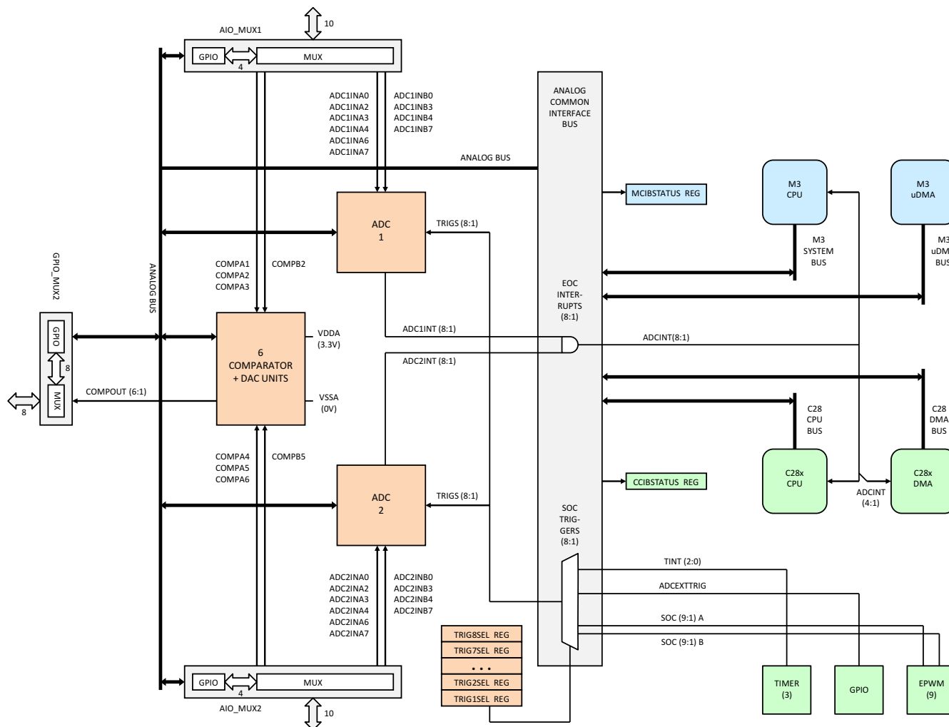
图 8-3. Analog Subsystem
