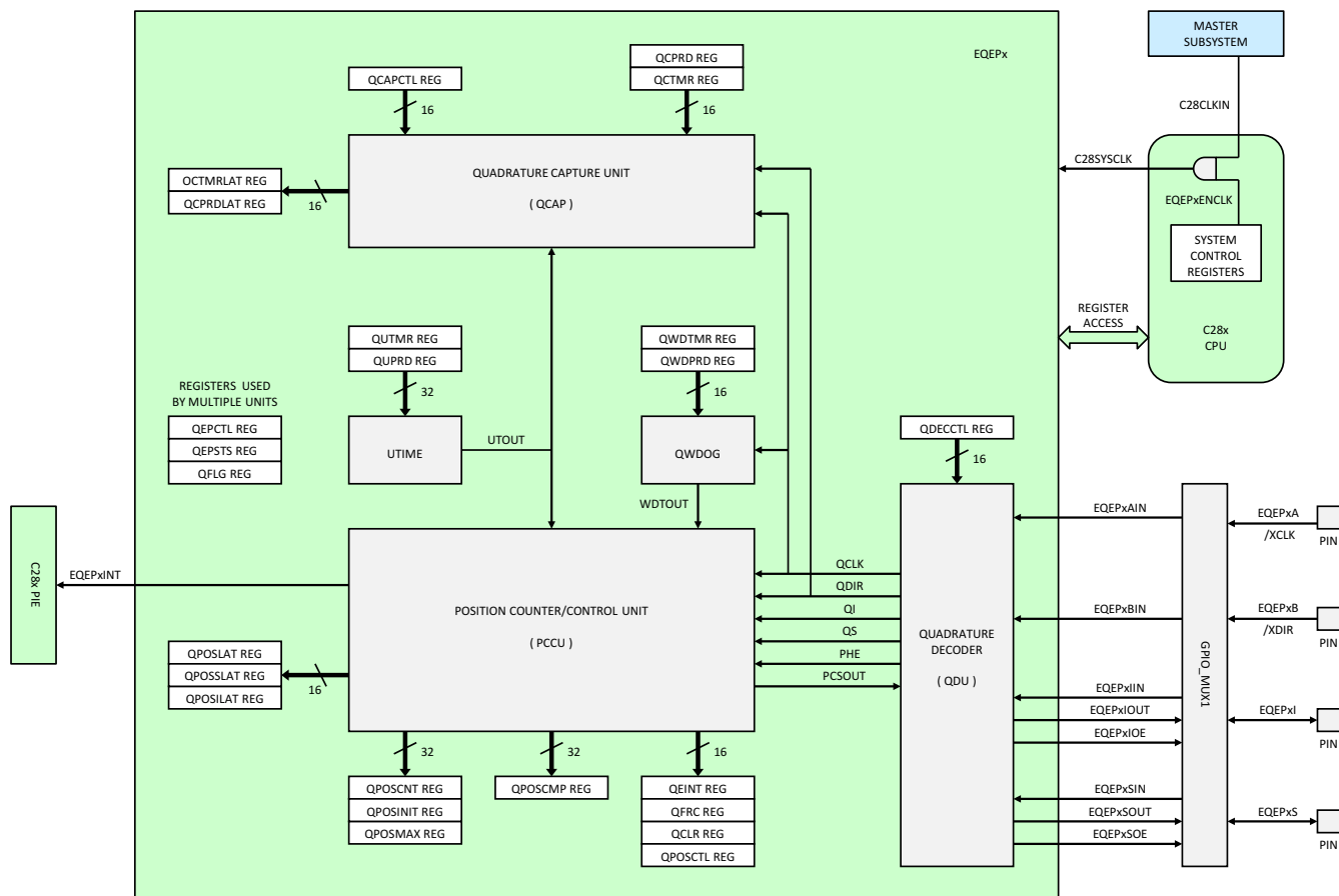
图 7-47. eQEP
