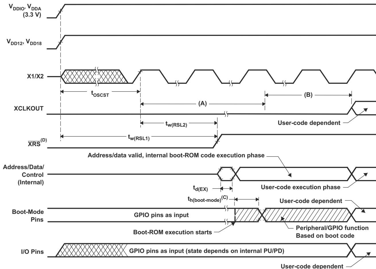
图 7-1. Power-On Reset
