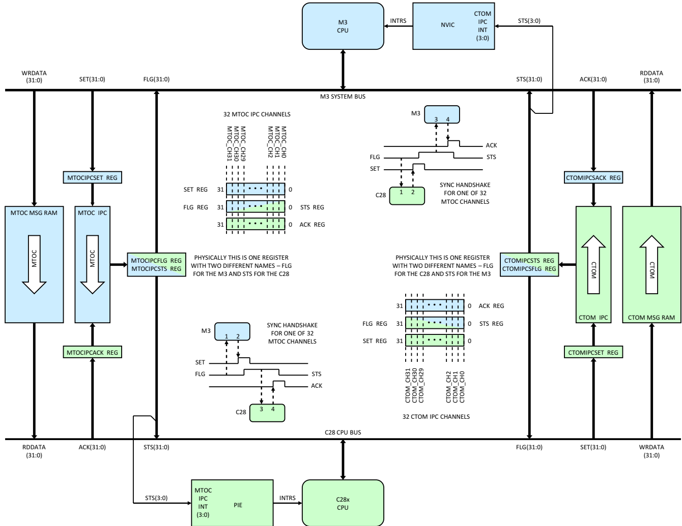
图 7-15. IPC
