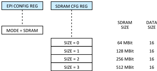
图 7-18. EPI SDRAM Mode
