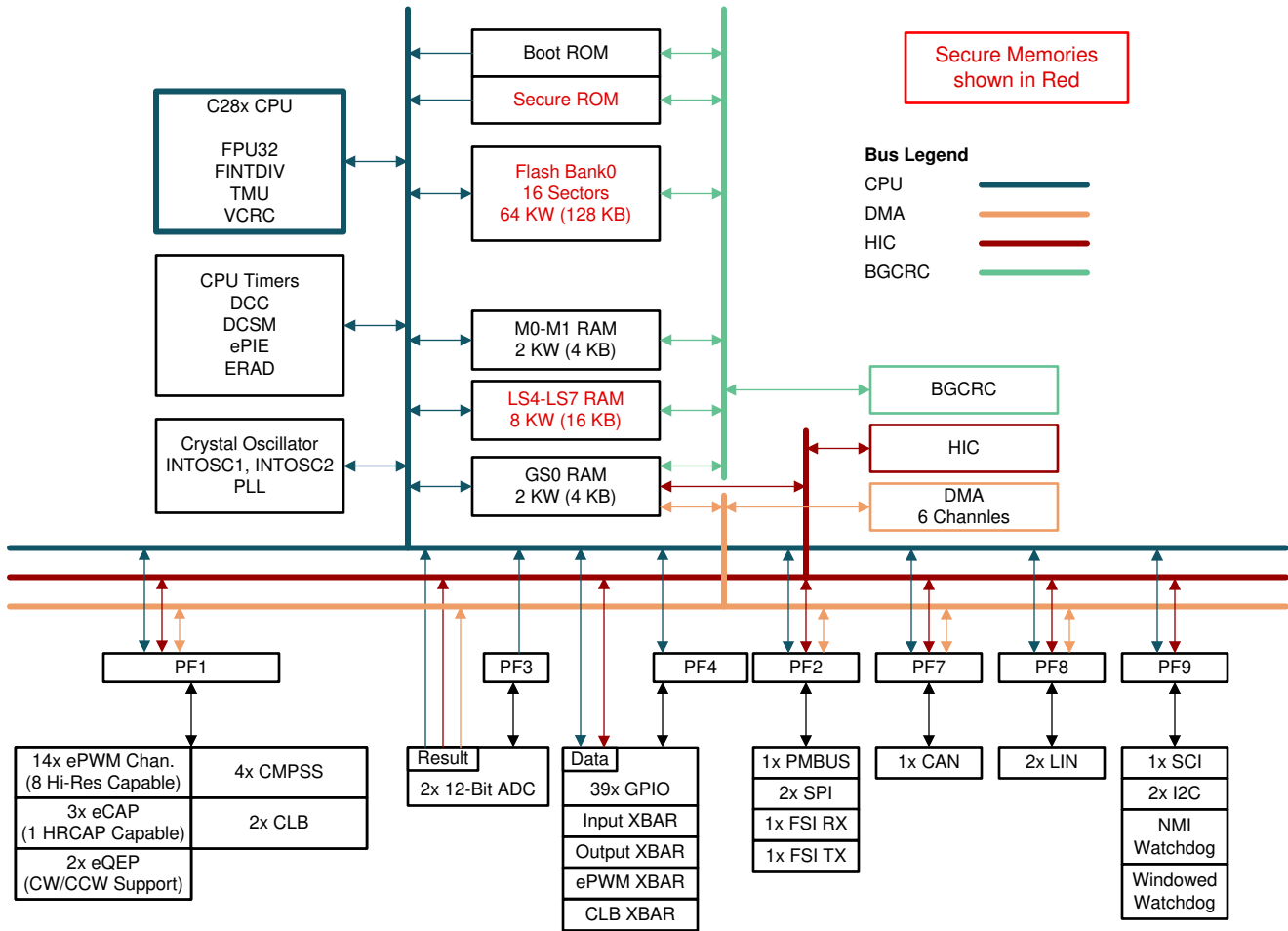
图 3-1. 功能方框图
