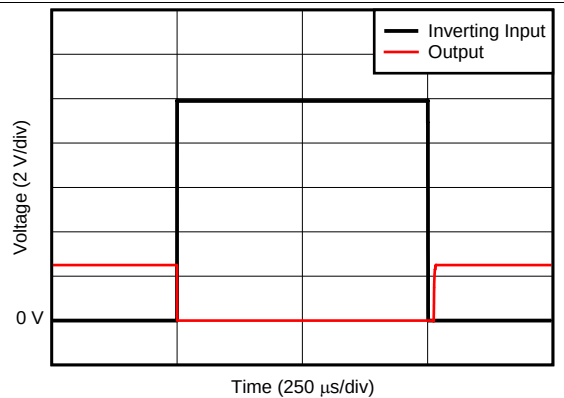
图 31. Step Response
