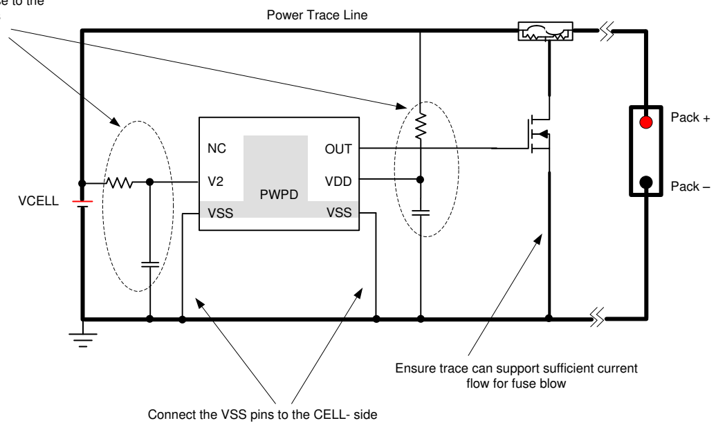
图 9-1. Layout Schematic
