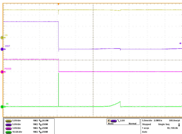
图 9-7. Output Hard Short-Circuit While ON
